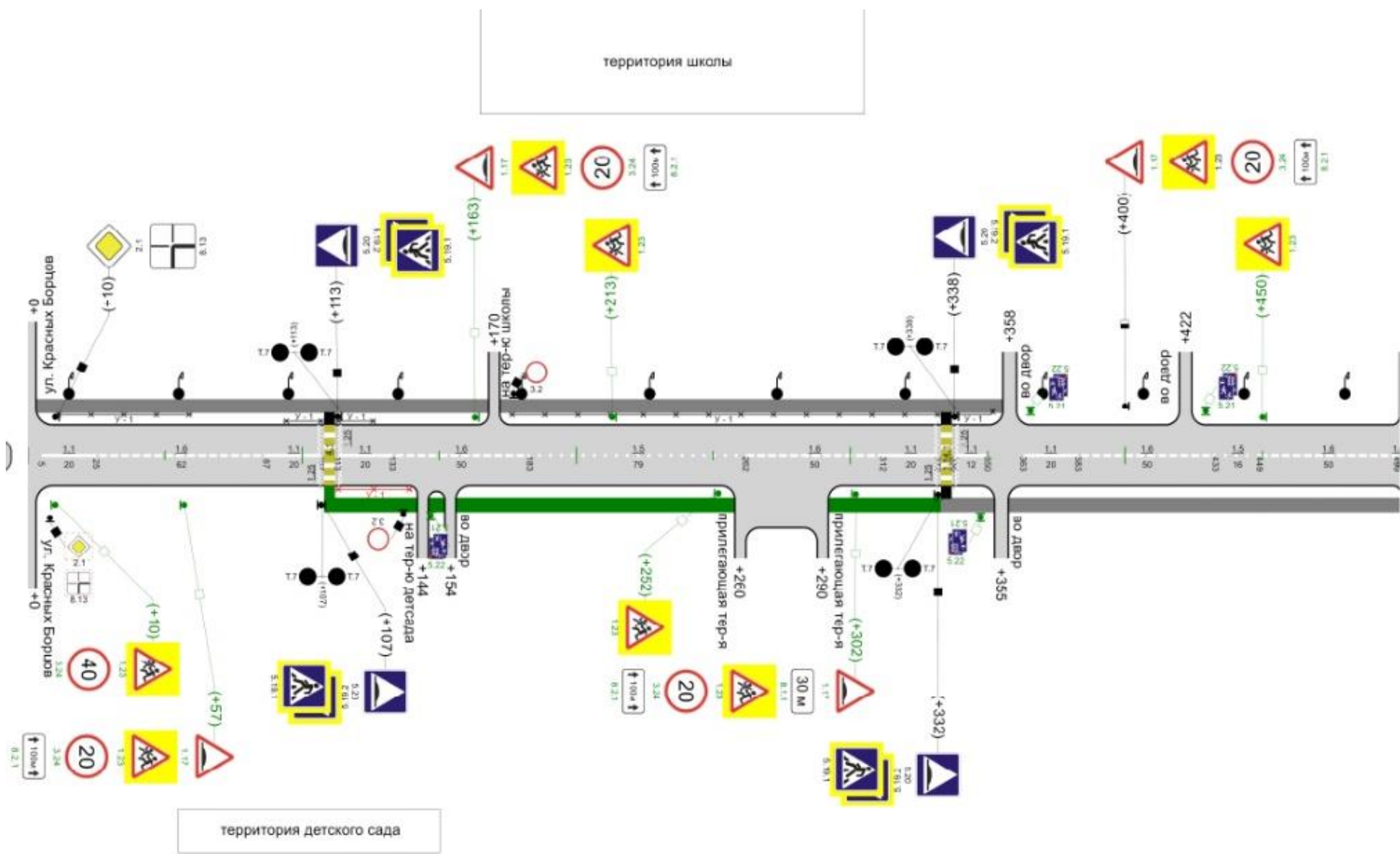
Схема 2 План-схема организации дорожного движения на улице Октябрьская
